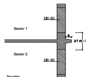
Figura 1.8 Encuentro forjado-fachada con saliente
